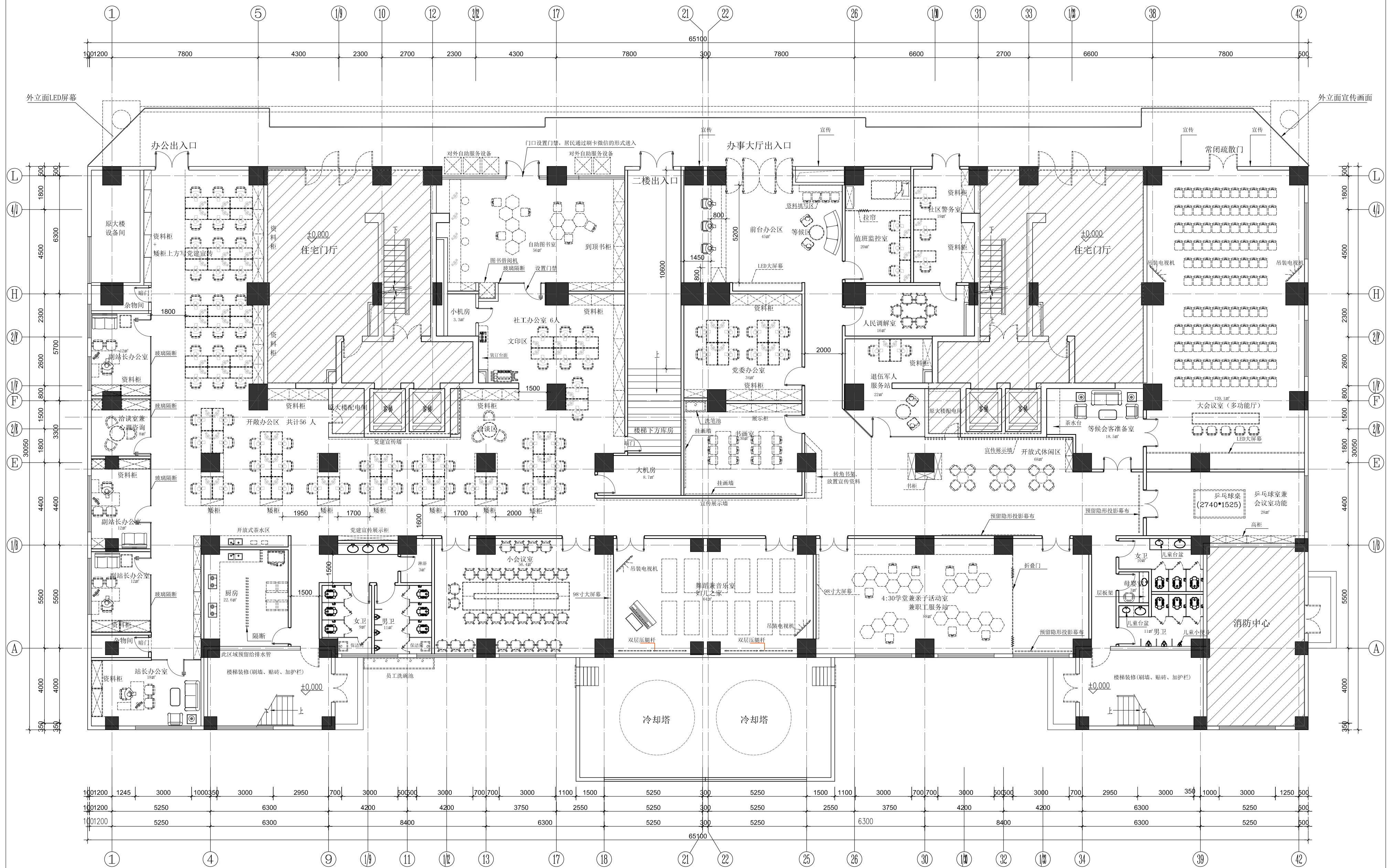
平面布置图 1:100
