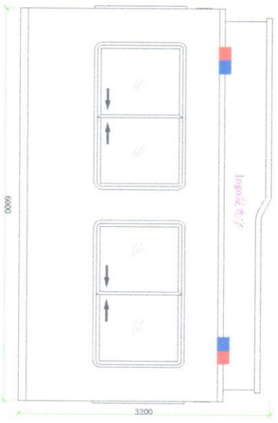
B立面图
