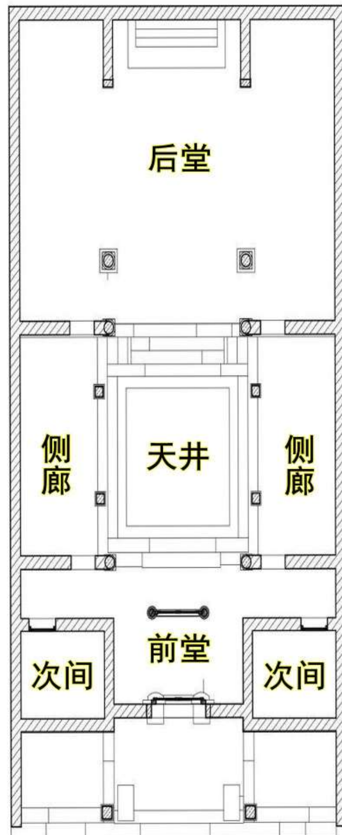
平面示意图
