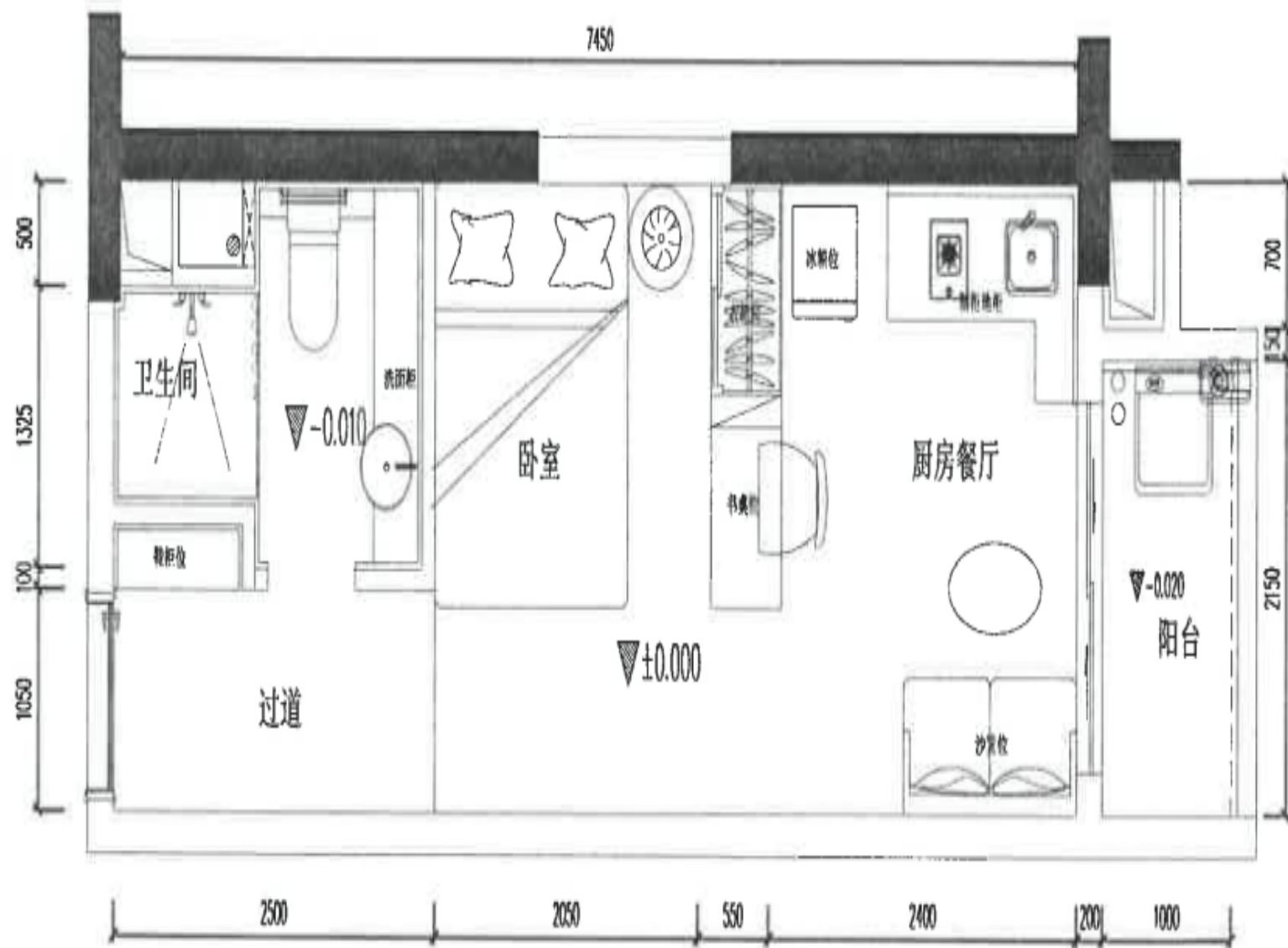
平面布置图
